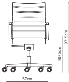
— 05/2A Depth 62cm Weight 15.3kg
